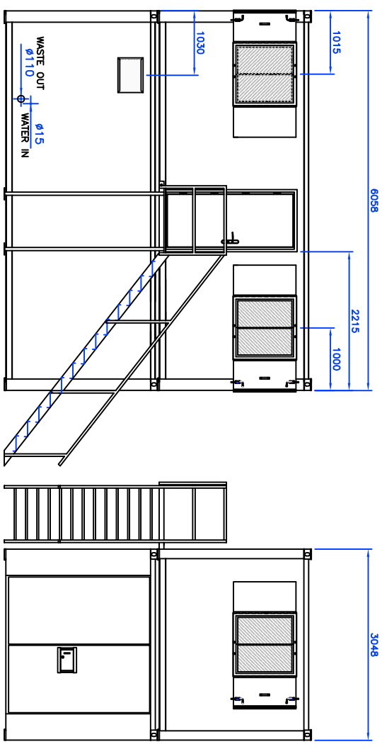
END ELEVATION
